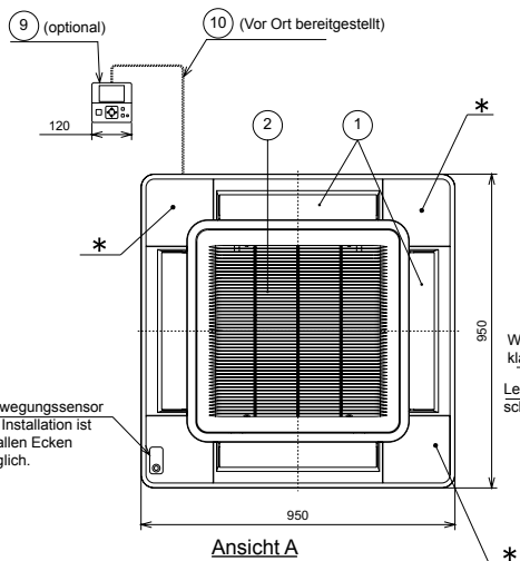
Separater Einbau
