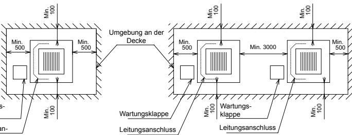
Geschlossener Einbau
